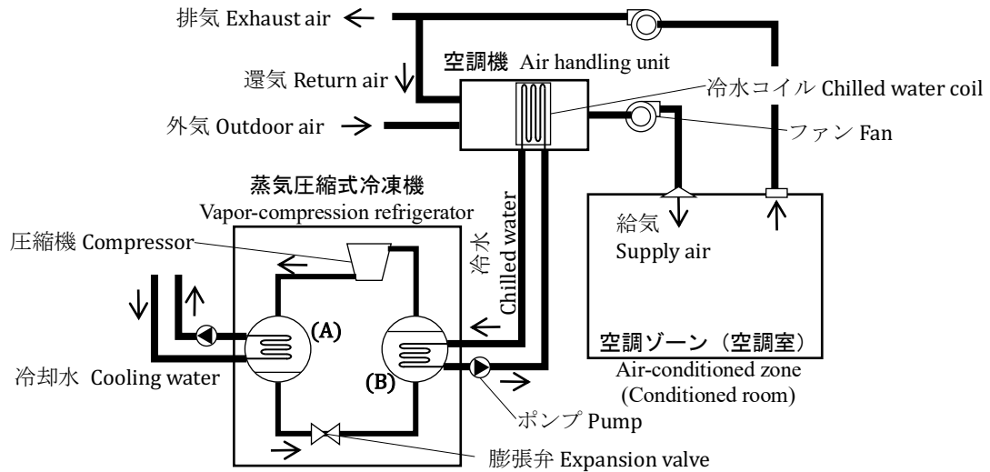
図 空調システム Figure: Air Conditioning System
