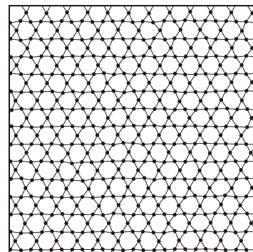
▲シミュレーションで形成されたカゴメ格子
