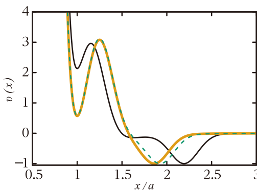
▲さまざまな粒子の相互作用
