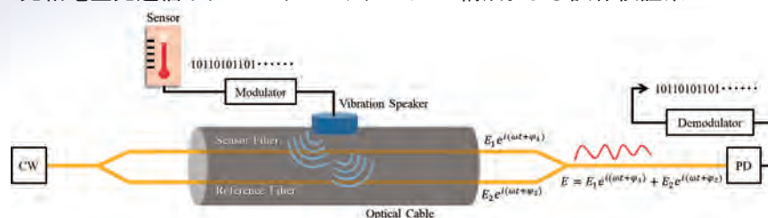
光ファイバケーブル外皮からの変調振動による屋外センサデータ伝送
