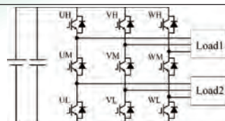
複数負荷駆動用インバータ
