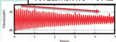
角度検出値を用いた 振動抑制制御システム
