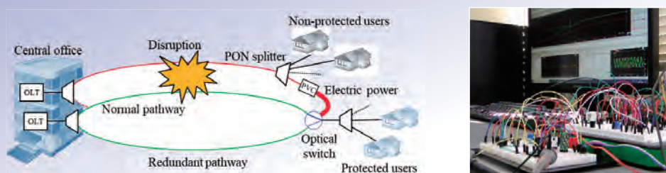
光給電型光通信ネットワークプロテクションの構成および試作検証系
