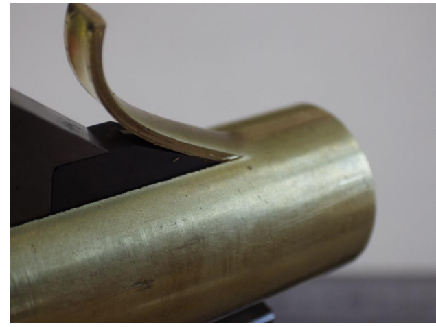
管材の切り粉レスな軸方向割断工法
