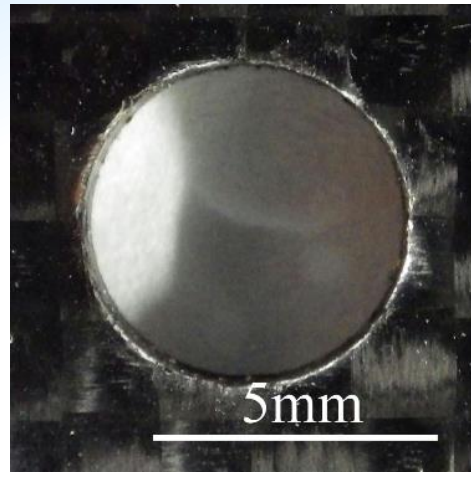
CFRTS板への穴あけ加工
