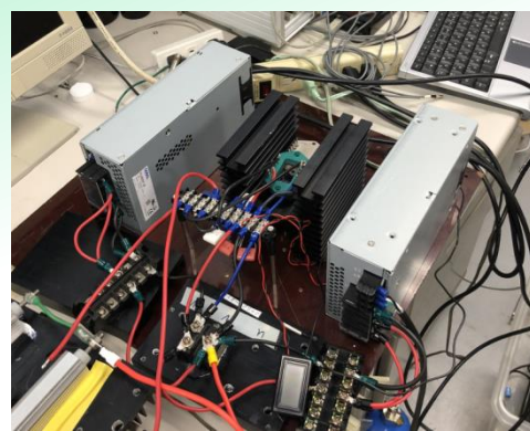
燃料電池模擬装置
