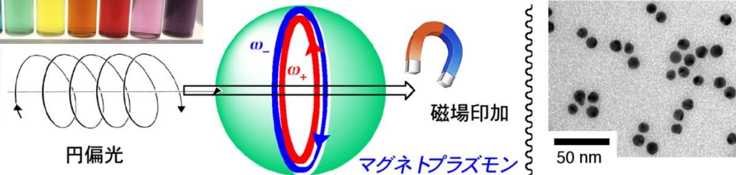
プラズモニック金属ナノ粒子分散液と磁気光学応答測定
