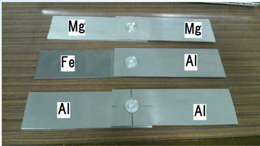
回転ツール点接合法による重ね継手
