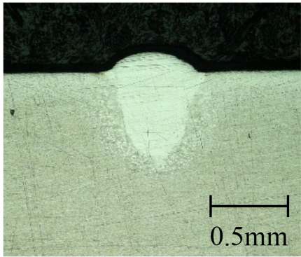
元素添加レーザー熔融硬化部 照射速度80mm/s
