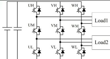
複数負荷駆動用インバータ
