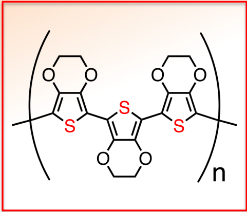
導電性ポリマー
