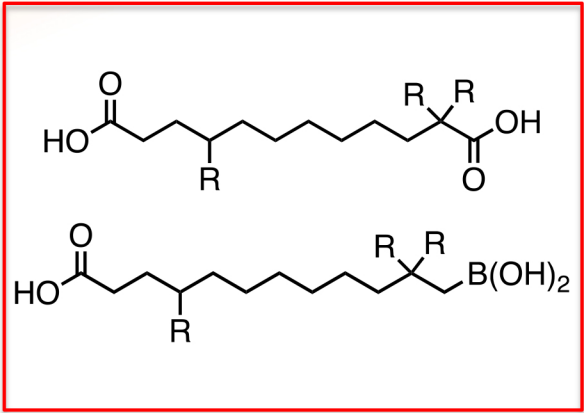
アルミ電解コンデンサ電解質
