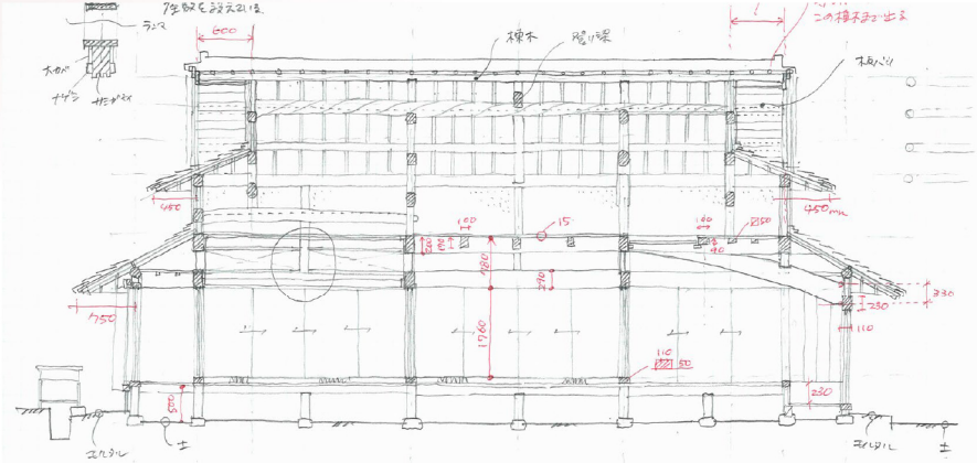
民家の実測調査の例
